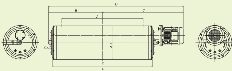
〈BMR-回転子外形図〉
