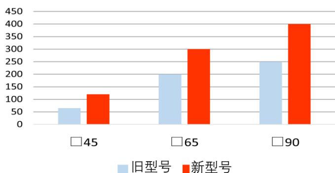
方形永磁座新旧型号吸附力比较
